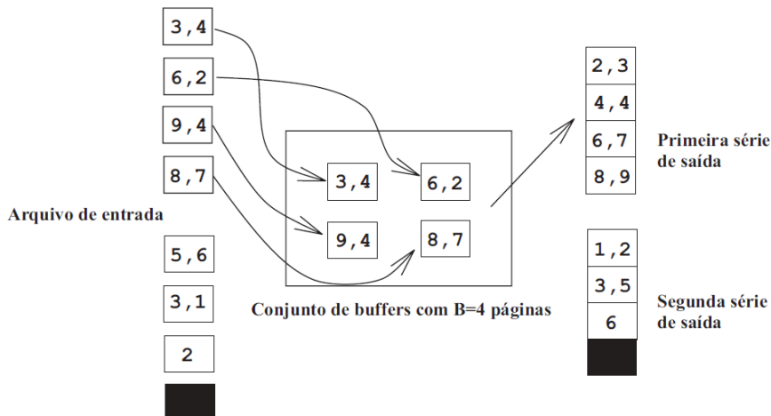
Figura 13.4 Merge-sort externo com B páginas de buffers: passagem 0.
