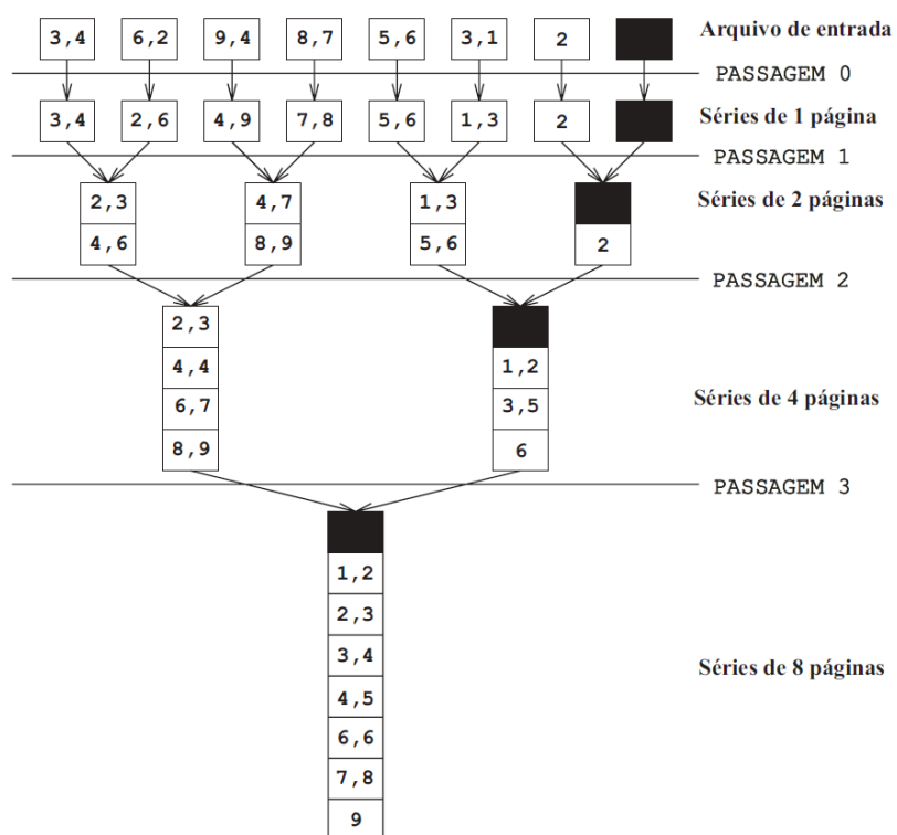
Figura 13.2 Merge-sort de duas vias de um arquivo de sete páginas.
