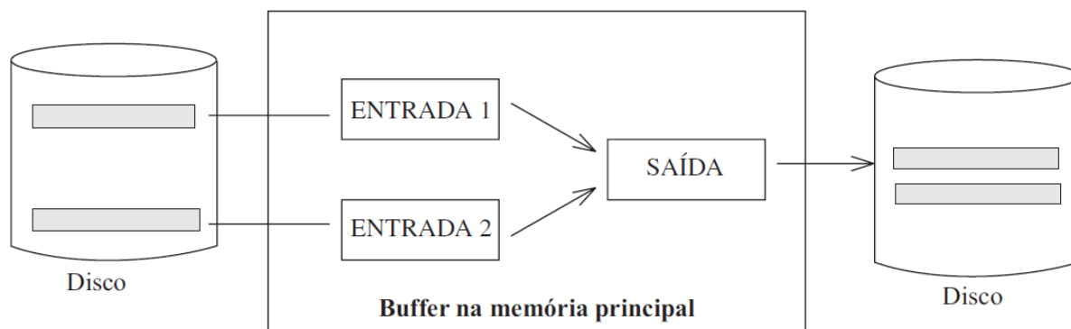
Figura 13.3 Merge-sort de duas vias com três páginas de buffer.
