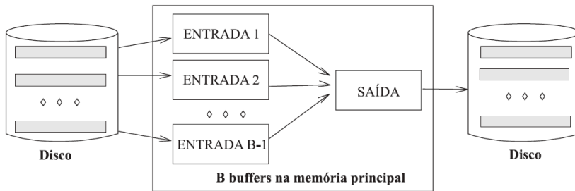
Figura 13.5 Merge-sort externo com B páginas de buffers: passagem i > 0 .
